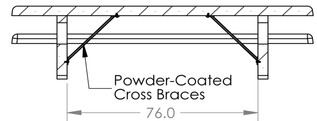
SECTION A-A SCALE 1 : 36
